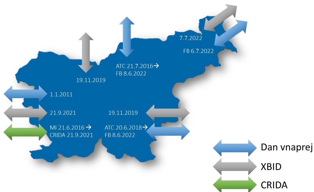
Slika 2: Regionalno spajanje trgov na mejah slovenskega elektroenergetskega sistema
